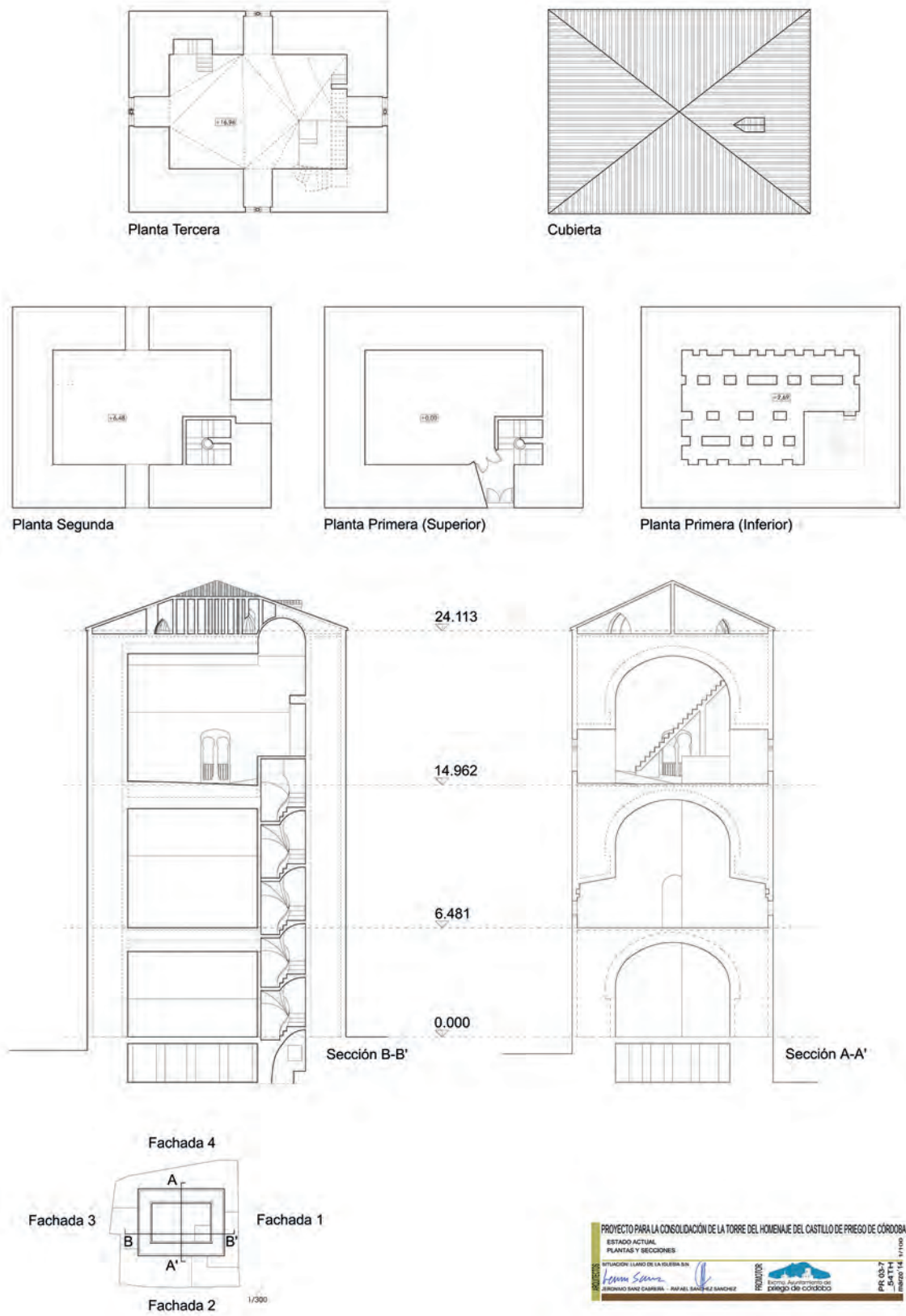
Fig. 5: Planimetría general de la torre con anterioridad al comienzo de los trabajos de consolidación, con indicación de Plantas y Fachadas referenciadas en el control arqueológico. Adaptada de la documentación incluida en el proyecto de consolidación firmado por los arquitectos Jerónimo Sanz y Rafael Sánchez.
