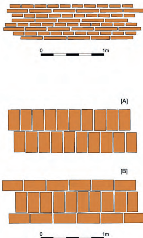
Fig. 61: Planta Segunda. Bóveda de ladrillo y despiece de la disposición latericia, con alternancia de A y B en el grueso de la rosca. Este mismo esquema se repite en la Planta Tercera.
